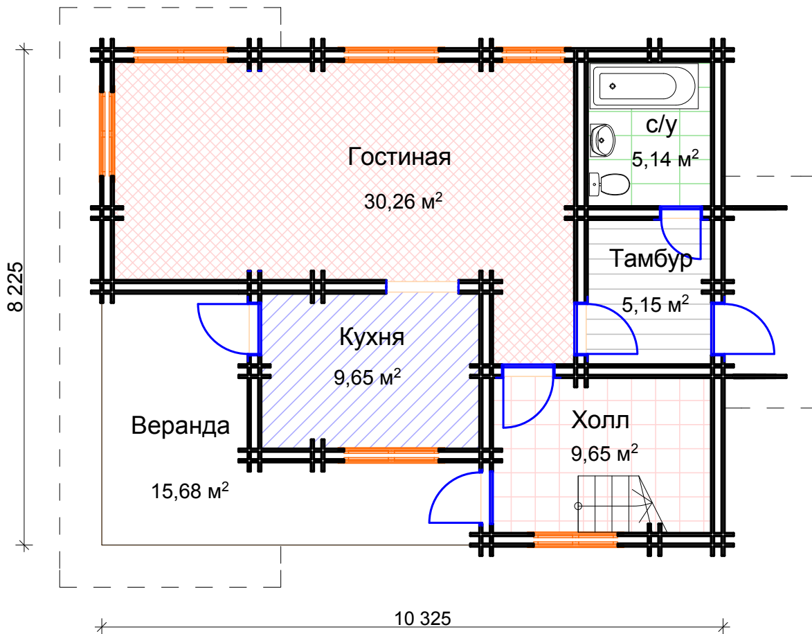
План помещений 1-ого этажа
